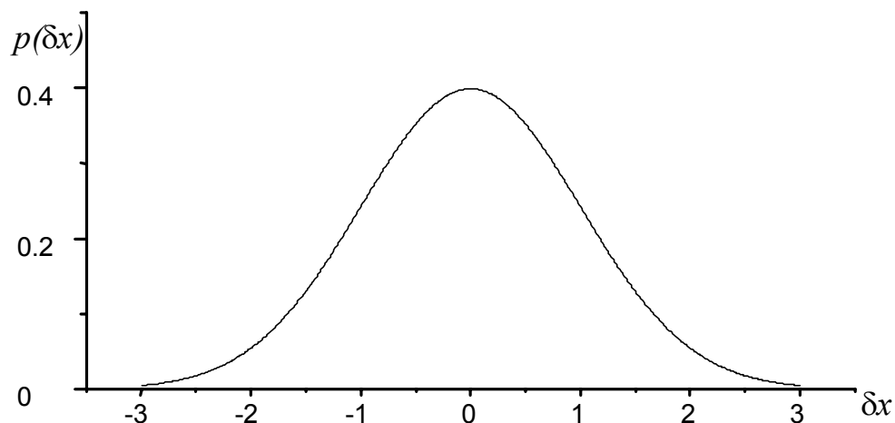
Рис.3. Функция Гаусса.
